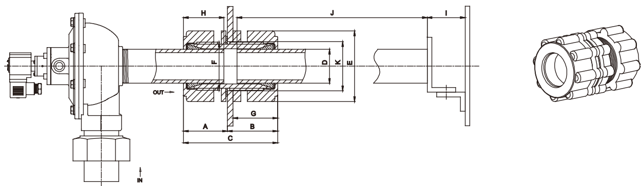
P2200G系列直角式电磁脉冲阀安装参考尺寸图
