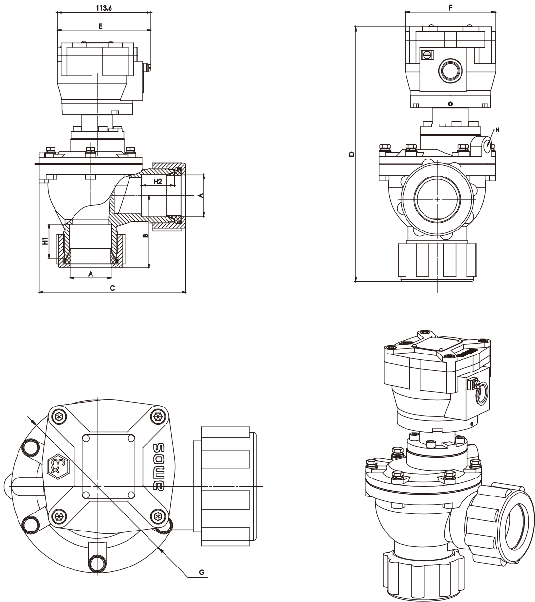
P2200T系列电磁脉冲阀外形尺寸图
