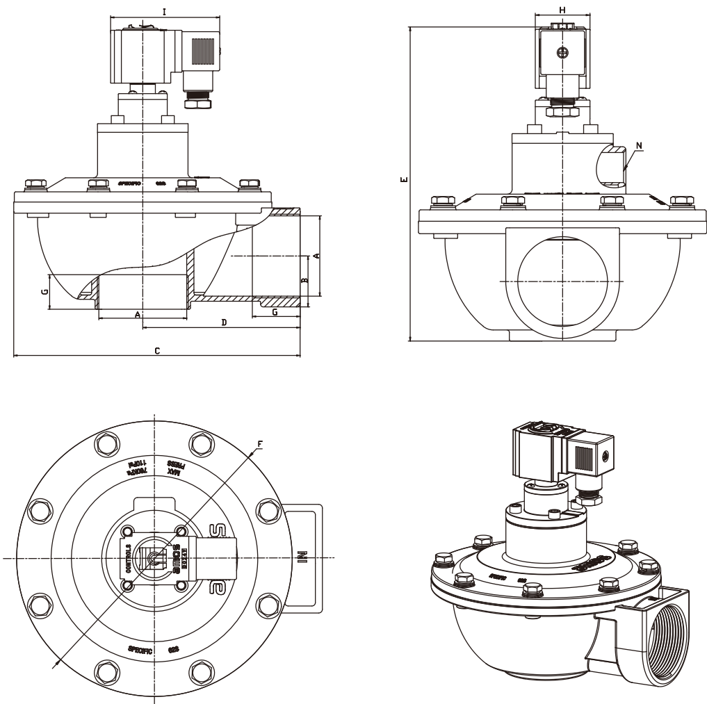
P2200G系列电磁脉冲阀外形尺寸图
