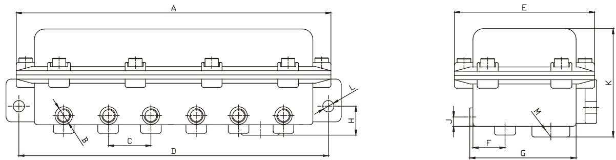
EV系列电磁阀先导盒外形尺寸图
