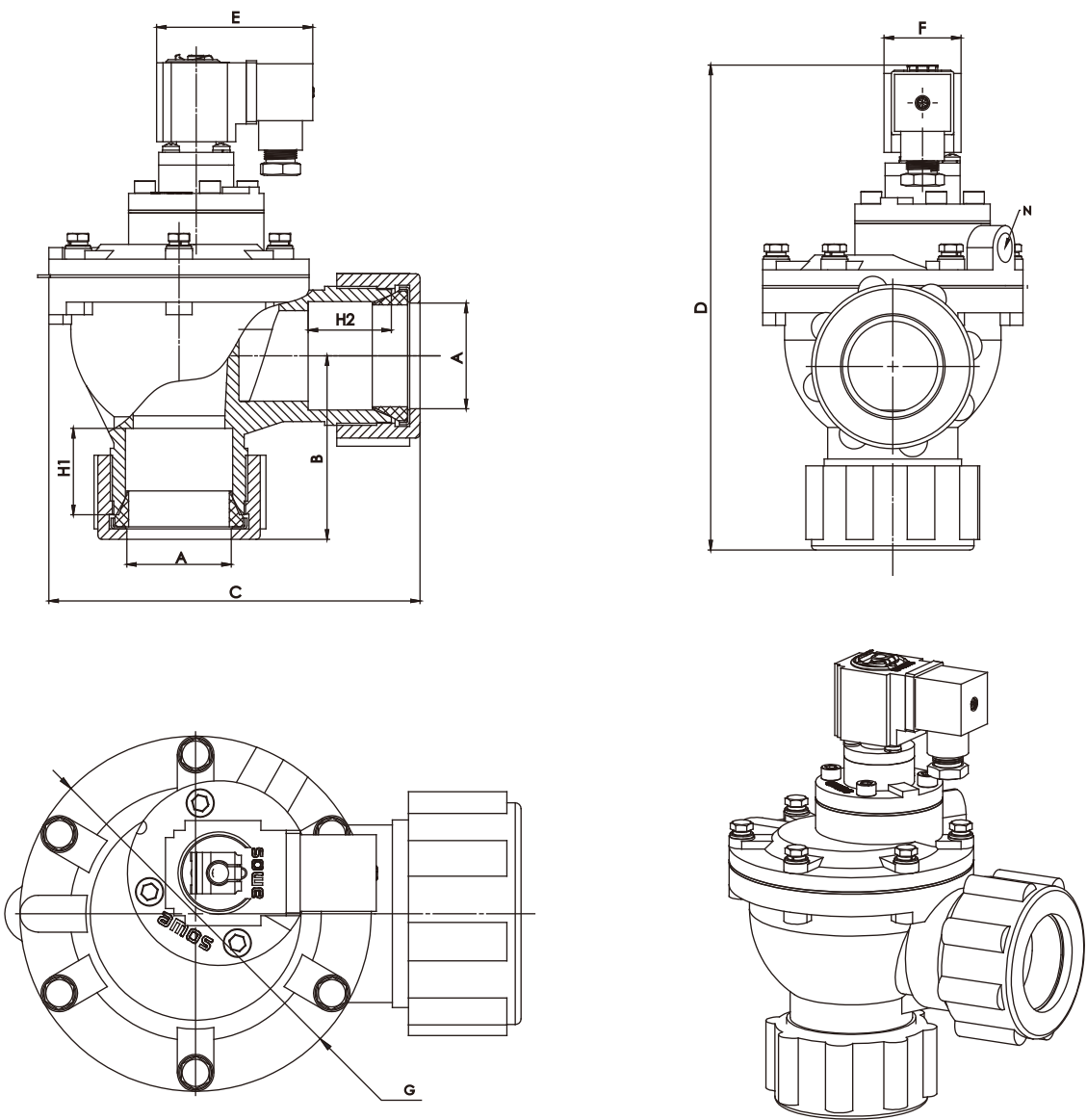
P2200T系列电磁脉冲阀外形尺寸图
